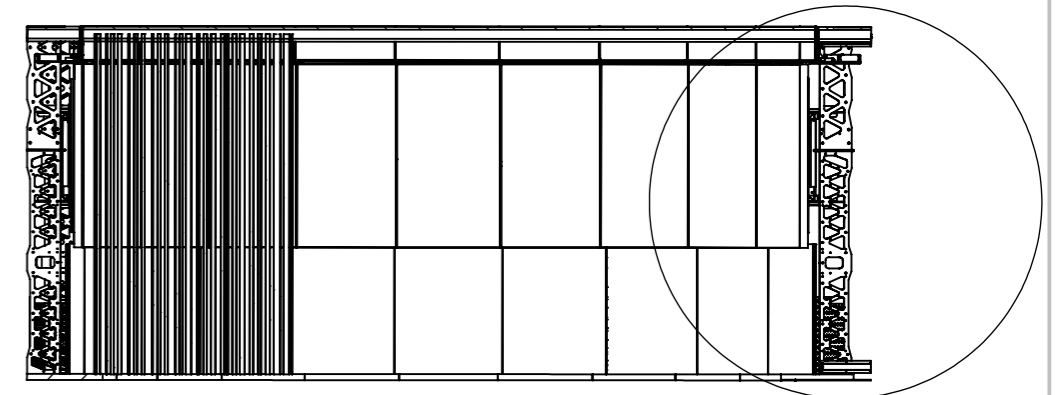
SECTION B-B C SCALE 1 : 50
